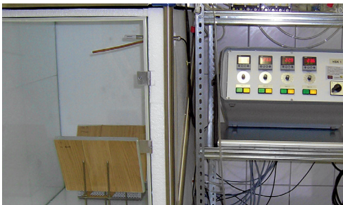
Bestimmung der Formaldehydemission
